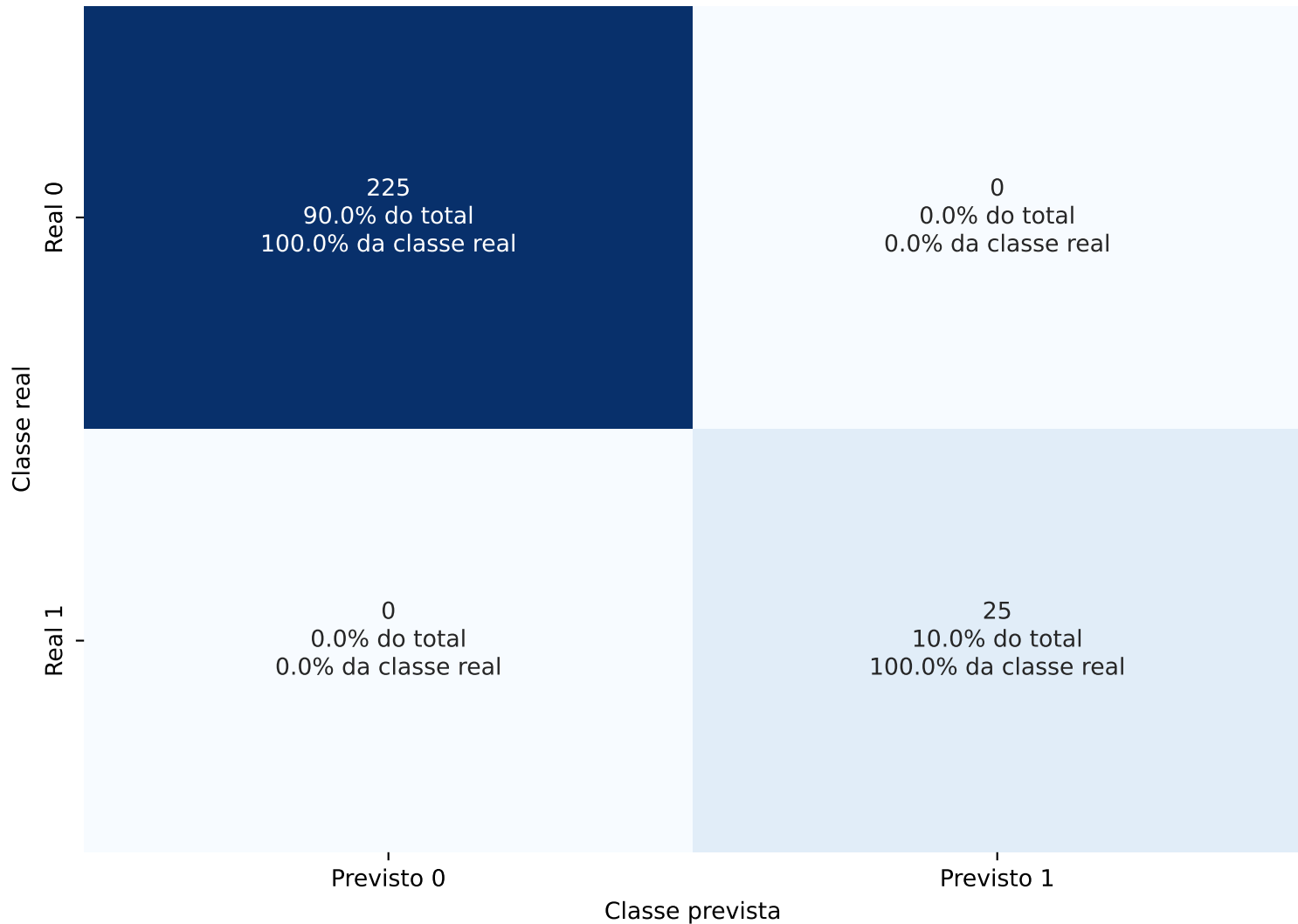
Matriz de Confusão — SVM_RBF_Balanced
